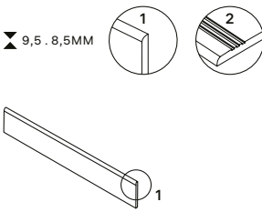
skirting plinthe sockel rodapé 8x60 NR MP-6170 8x90 NR MP-6260 8x120 NR MP-6260
