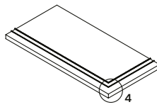
* step tread "L" corner inox nez de marche "L" angle inox ecke stufenplatte "L" inox degrau "L" canto inox 30x60 NR . A MP-6650 30x120 NR . A MP-6710
