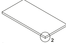
* step tread "L" corner nez de marche "L" angle ecke stufenplatte "L" degrau "L" canto 30x60 NR . A . ASR MP-6630 30x90 NR . A . ASR MP-6645 30x120 NR . A MP-6655
