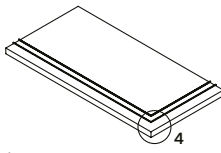
* step tread "L" corner inox nez de marche "L" angle inox ecke stufenplatte "L" inox degrau "L" canto inox 30x60 NR . A MP-6650 30x90 NR . A MP-6690 30x120 NR . A MP-6710
